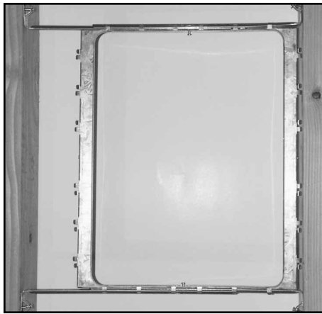
The NCB-M-WM "hole saving" bracket fits in between the studs, so there is no bulge in the drywall. / L'appui de nouvelle construction (NCB-M-WM) s'adapte entre les goujons, tellement là n'est aucun bombement dans le plaques de plâtre.
